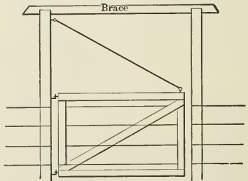
FIG. 102.—Gate tie.
