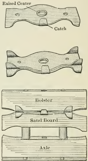
FIG. 144.—Bolster plates.
