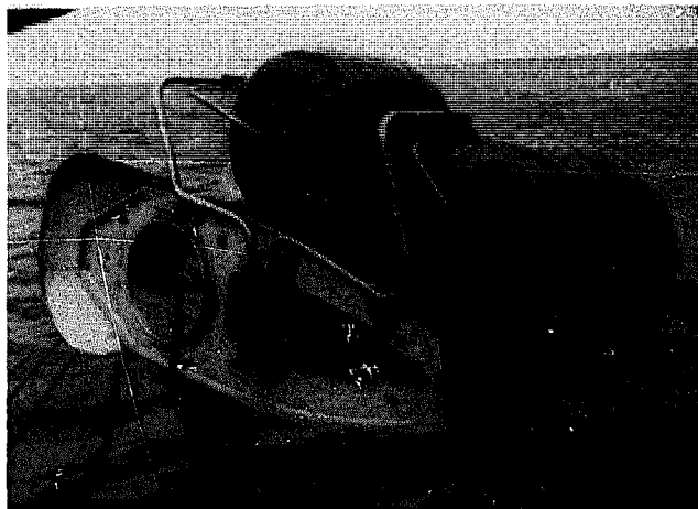
Fig 689 Danish automatic gillnet hauler. (Courtesy of Grenaa Smedie og Maskinfabrik, Grenaa, 1979).
